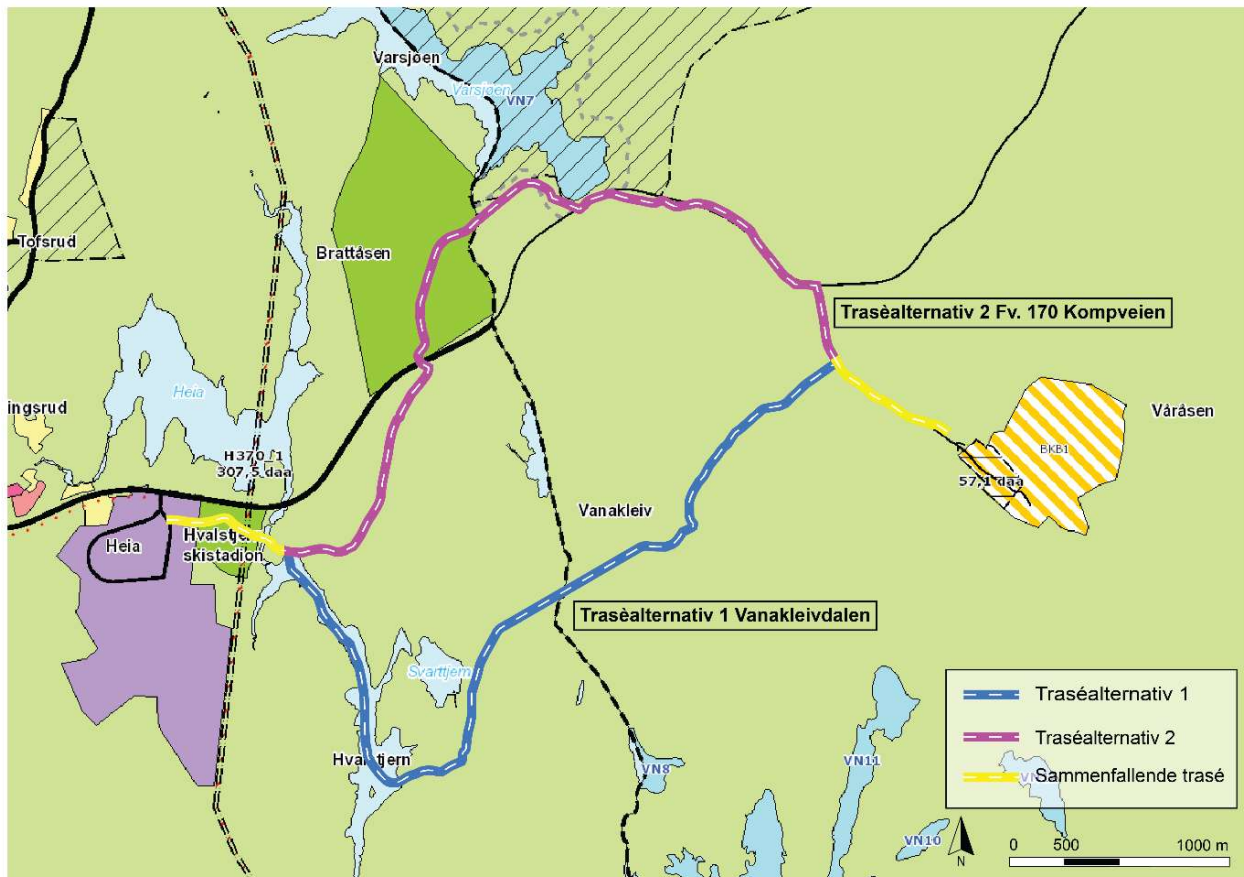
Figur 2: Gjeldende kommuneplan og de to traséalternativene. Alternativ 1 gjennom Vanakleivdalen markert med blå linje og alternativ 2 langs fv. 170 Kompveien markert med rosa linje. Gul linje markerer strekningene der traséene er sammenfallende.
